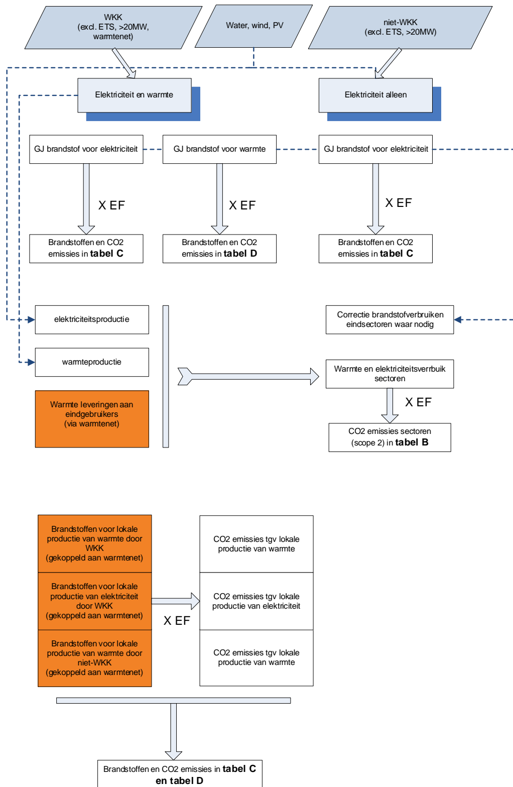
Figuur 16: Schematisch overzicht van input, berekeningen en output voor de sector lokale energieproductie
