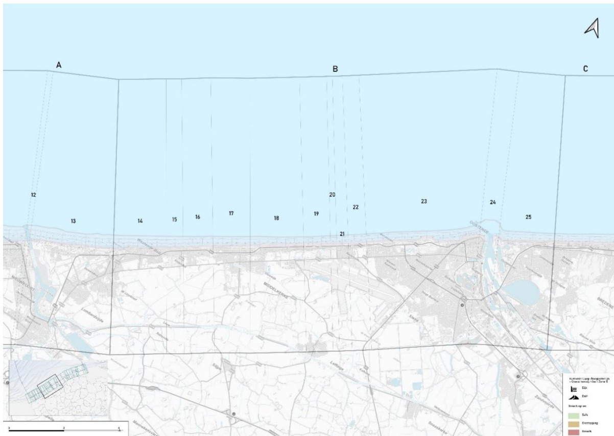
Kaart I-6: Overzicht kustvakken met overtopping of doorbraak van de dijk voor +2 m zeespiegelstijging voor de Middenkust-West.
