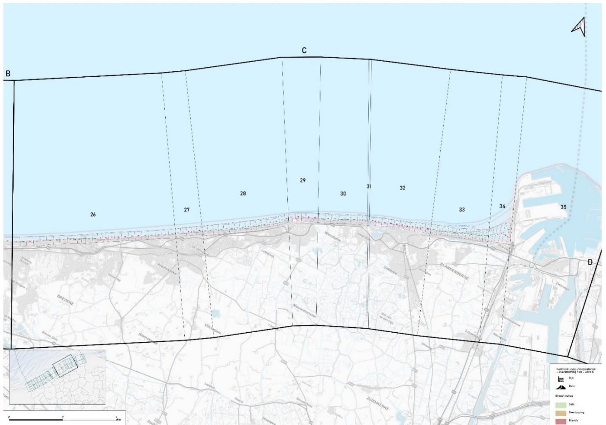
Kaart I-11: Overzicht kustvakken met overtopping of doorbraak van de dijk voor +3 m zeespiegelstijging voor de Middenkust-Oost.
