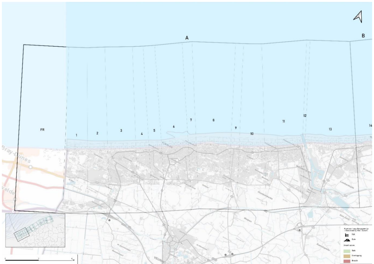
Kaart I-5: Overzicht kustvakken met overtopping of doorbraak van de dijk voor +2 m zeespiegelstijging voor de Westkust.
