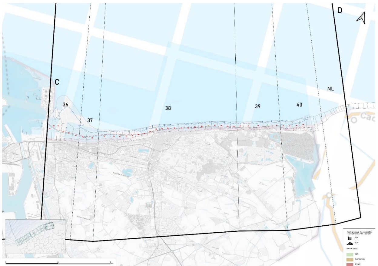
Kaart I-12: Overzicht kustvakken met overtopping of doorbraak van de dijk voor +3 m zeespiegelstijging voor de Oostkust.
