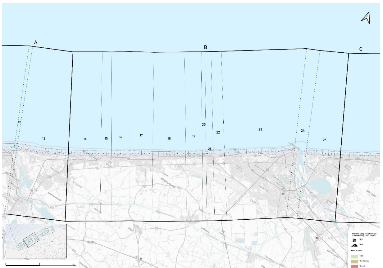
Kaart I-10: Overzicht kustvakken met overtopping of doorbraak van de dijk voor +3 m zeespiegelstijging voor de Middenkust-West.
