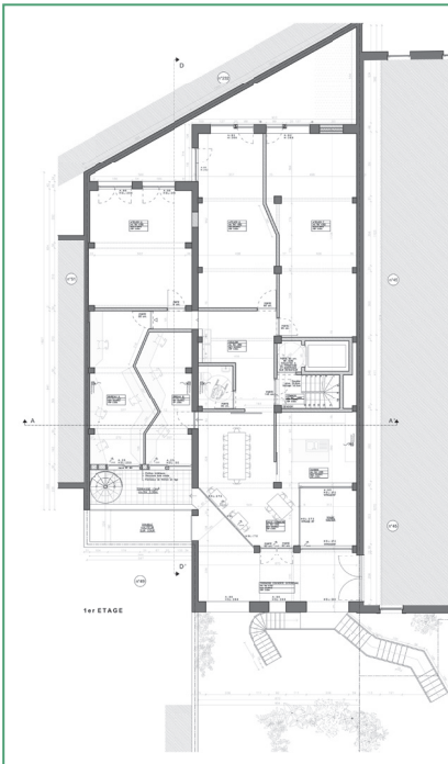
Grondplan 1 e verdieping © Lhoas&Lhoas Architectes
