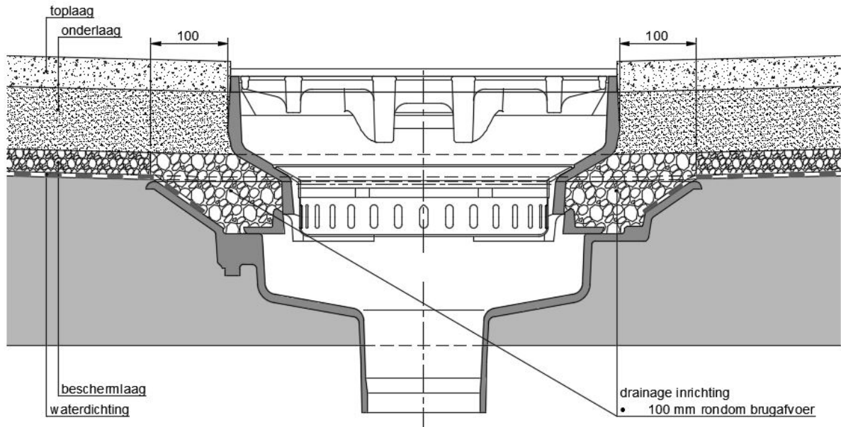
Figuur 32-21-5: Straatkolck voorzien van een extra inlaat op het niveau van de afdichting
