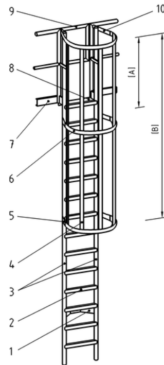
Figuur 21-5-13: Vaste ladder met kooi
