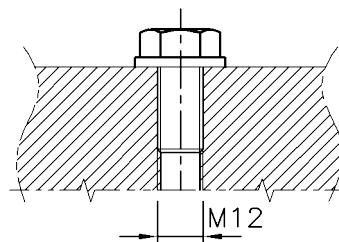
Figuur 32-10-22: type VII-2
