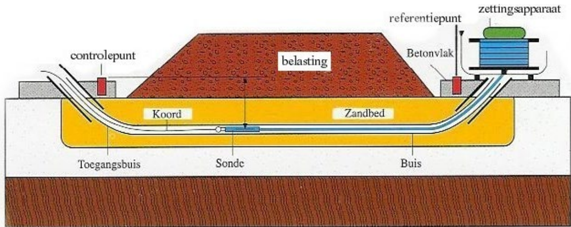
Figuur 22-2-13: De methode met het hydrostatisch zettingsapparaat
