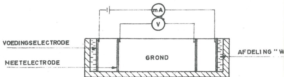
Figuur 24-4-2: Uitrusting voor metingen met gelijkstroom
