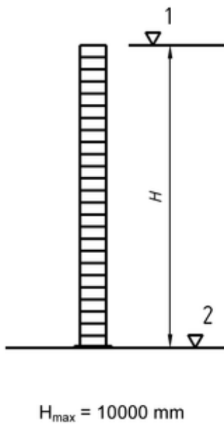
Figuur 21-5-11: Vaste ladder zonder rustplatform, zonder kooi
