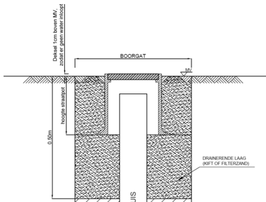
Figuur 22-2-11: Afwerking d.m.v. een straatpot – gefundeerd in een drainerende laag
