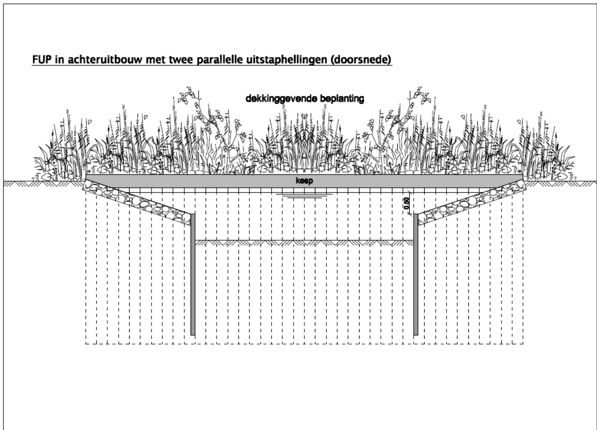
Figuur 21-5-8: Fup in achteruitbouw met twee parallelle uitstaphellingen (doorsnede)
