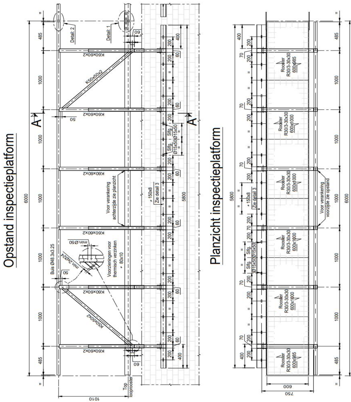
Figuur 32-34-1: Principe opstand en planzicht inspectieplatform
