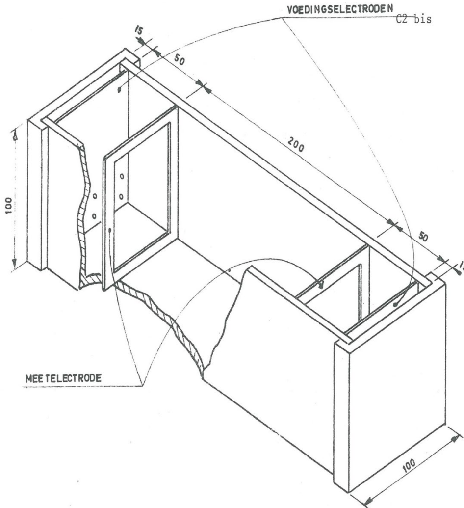
Figuur 24-4-1: Resistiviteitscel voor metingen met gelijkstroom (afmetingen in mm)
