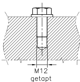
Figuur 32-10-23: type VII-3
