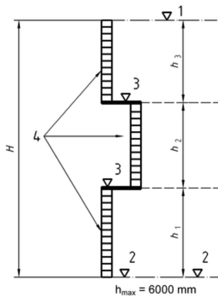
Figuur 21-5-12: Vaste ladder zonder kooi met verspringen ter plaatse van de rustplatformen
