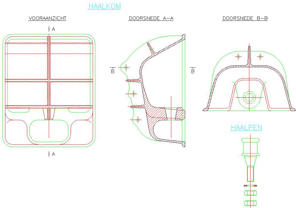
Figuur 32-62-1: Schematische voorstelling van een haalkom met demonteerbare haalpen
