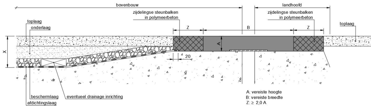
Figuur 32-31-8: Inbouw flexibele voegovergang o.b.v. polymeren – nieuwbouw
