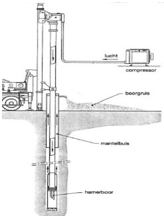
Figuur 22-2-5: Hamerboren
