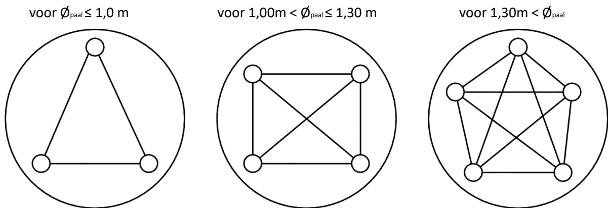
Figuur 24-1-1: schikking PVC buizen in boorpalen voor CSL-metingen
