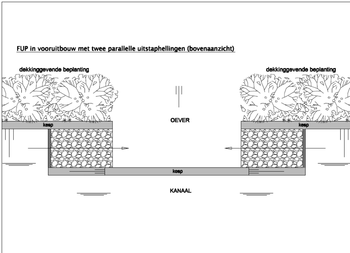
Figuur 21-5-3: Fup in vooruitbouw met twee parallelle uitstaphellingen (bovenaanzicht)
