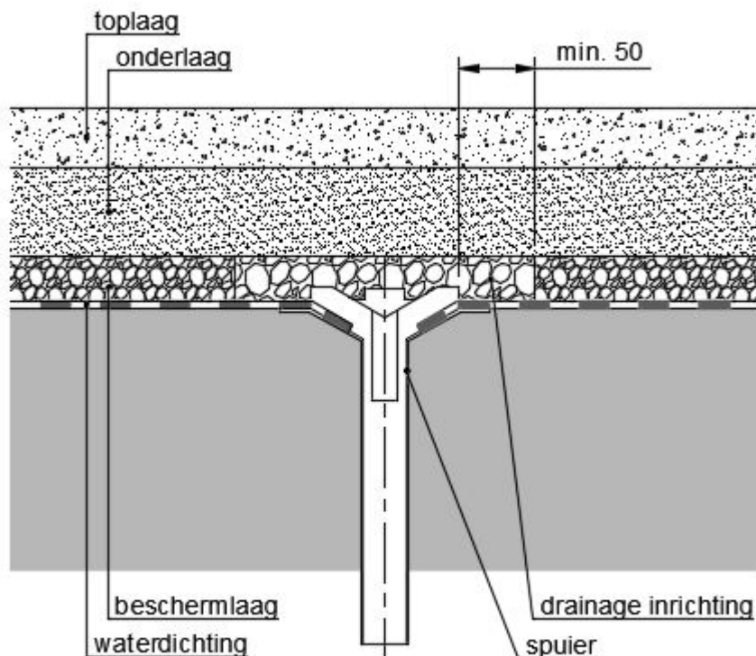
Figuur 32-21-6: ingestorte spuiër met voldoende drainage aan alle inlaten
