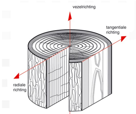
Figuur 30-1-1: Hoofdvlakken of zaagwijzen in het hout
