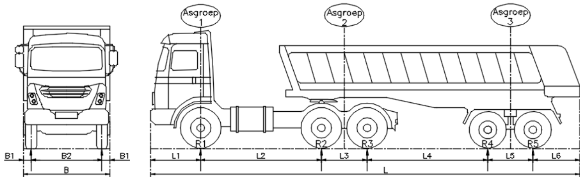
Figuur 35- 1-2: Het typevoertuig 1 van 43ton
