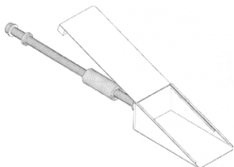
Figuur 22- 2-6: Bodemschep
