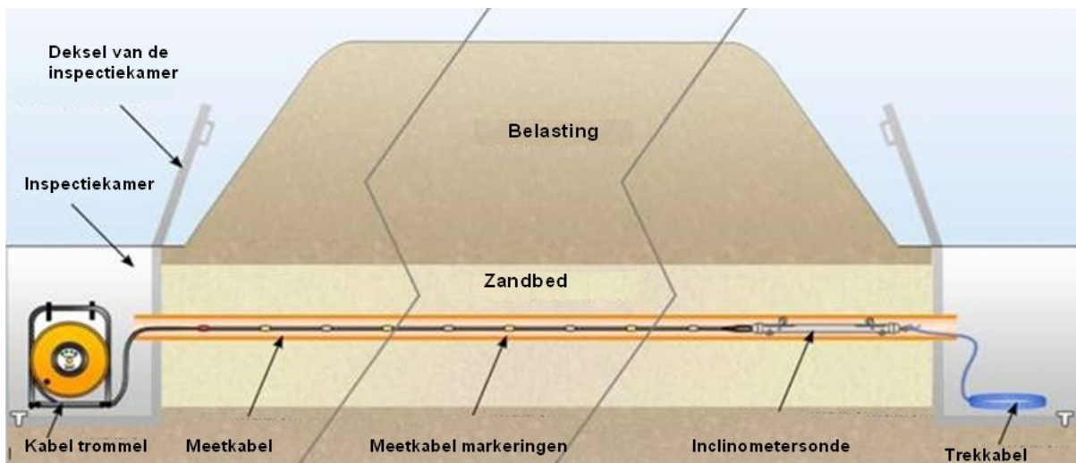
Figuur 22-2-14: De methode met de horizontale inclinometersonde
