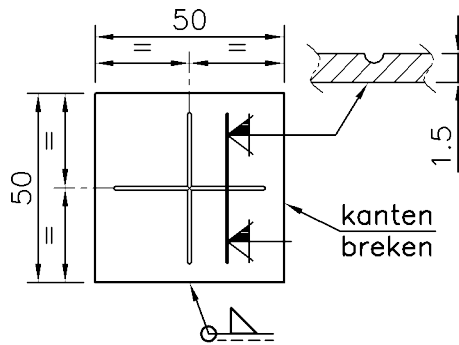
Figuur 32-10-25: type VIII
