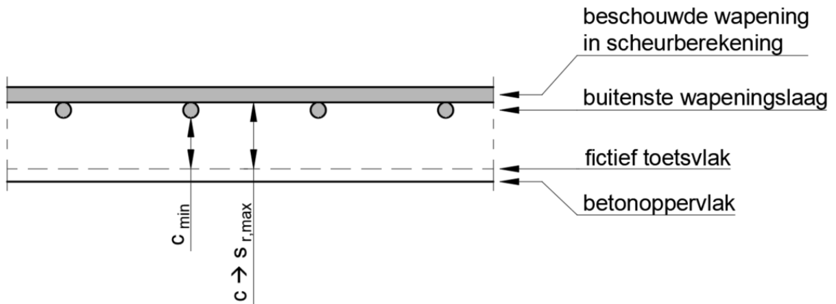
Figuur 21-6-4: Duiding bij berekening scheurwijdte
