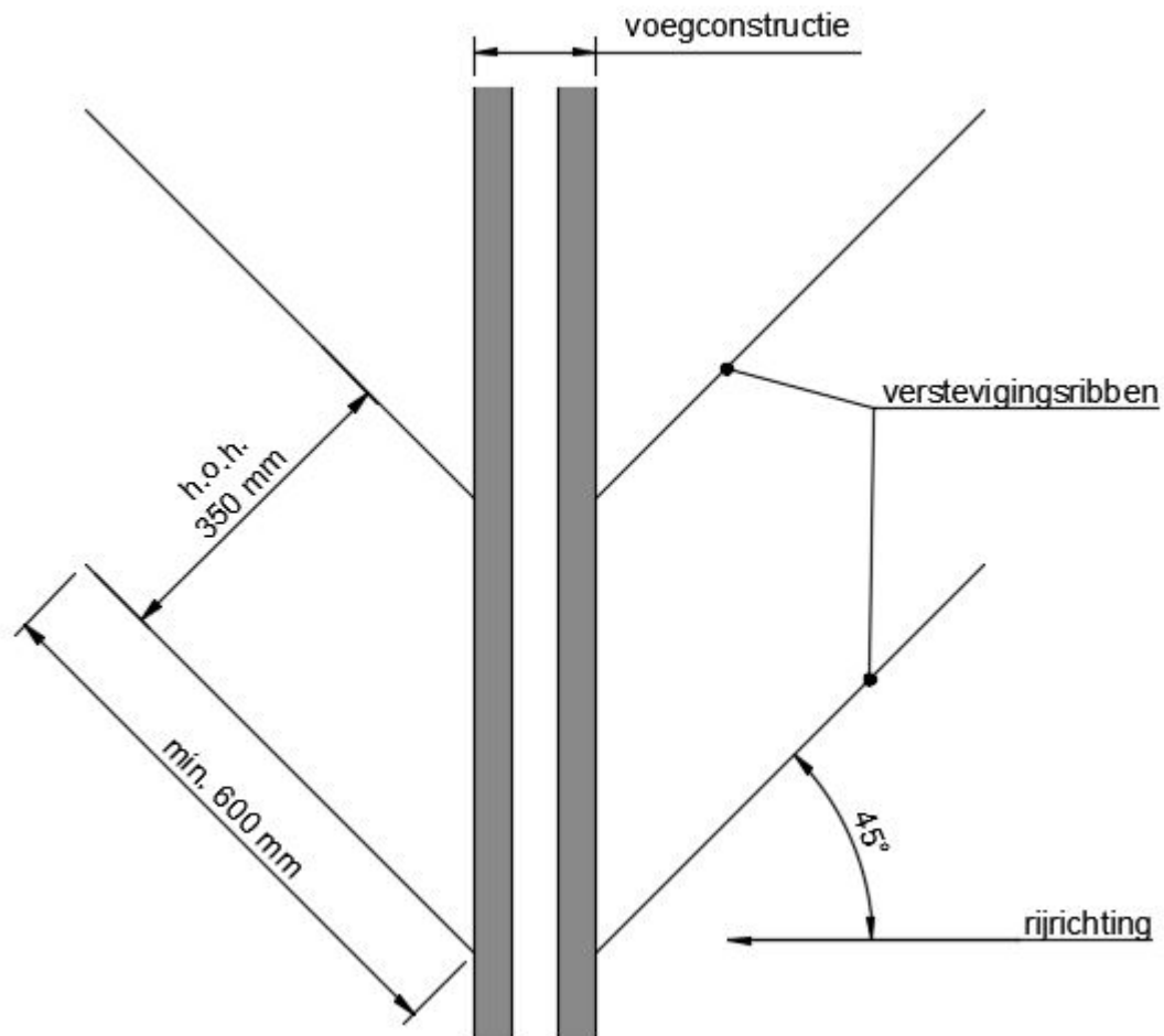
Figuur 32-31-10: Principe verstevigingsribben
