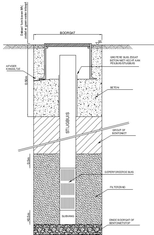
Figuur 22-2-10: Afwerking d.m.v. een straatpot – afwerking in beton
