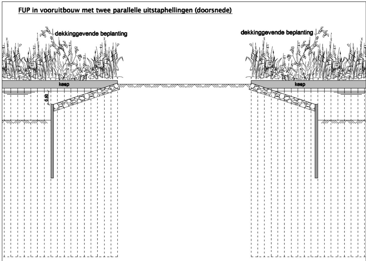
Figuur 21-5-4: Fup in vooruitbouw met twee parallelle uitstaphellingen (doorsnede)
