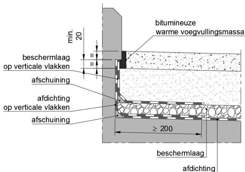
Figuur 32-21-4: typedetail uitsparingen en afschuiningen
