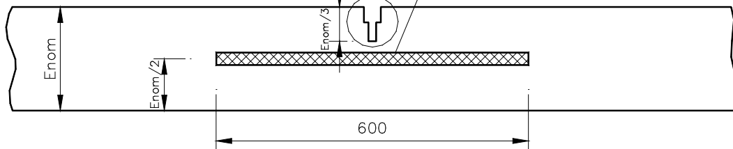
Figuur 6-10-5: Doorsnede A – A' (alle maten in mm) - dwarse krimpvoeg type 1: met zaagsnede en sponning met voegvulling
