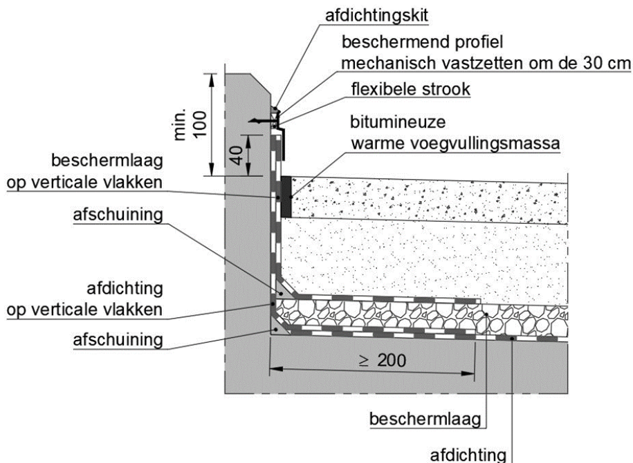
Figuur 32-21-3: Typedetail beschermend profiel
