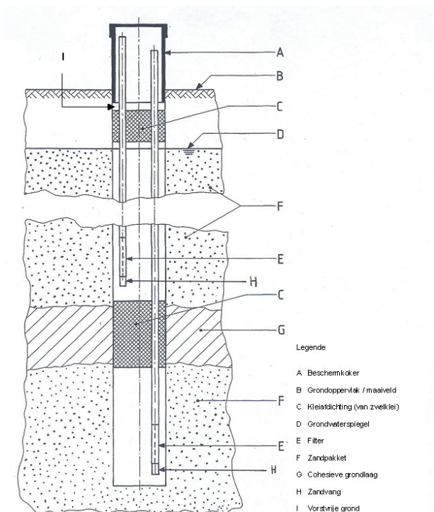
Figuur 22-2-12: Afwerking d.m.v. een beschermkoker en opbouw meerdere peilbuizen in één boorgat.
