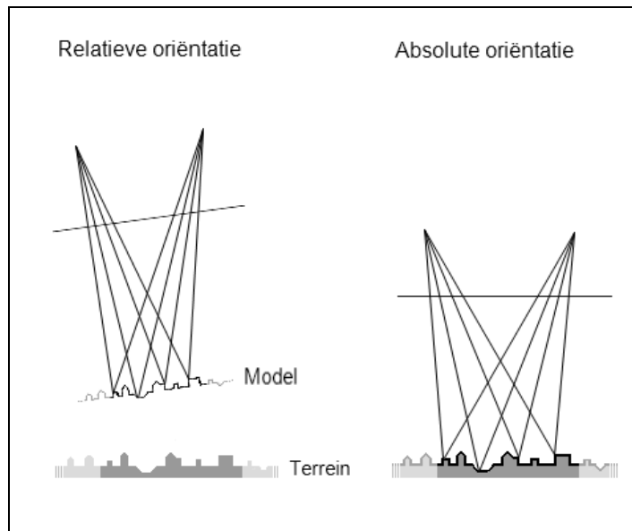
Figuur 1 : opeenvolgende stappen van de aerotriangulatie (de relatieve oriëntatie) en de blokvereffening (de absolute oriëntatie)
